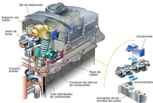
Sección de la culata y órganos internos
